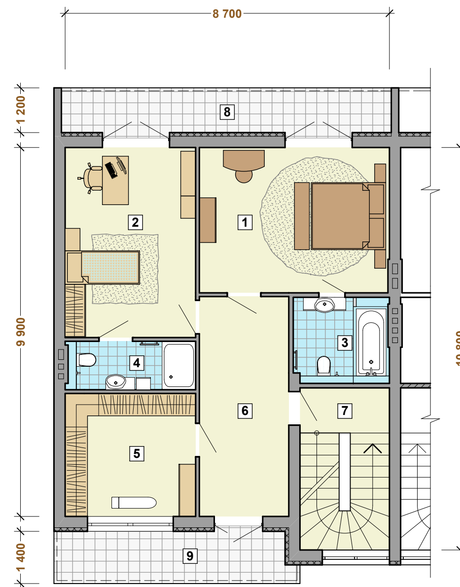
ВТОРОЙ ЭТАЖ
