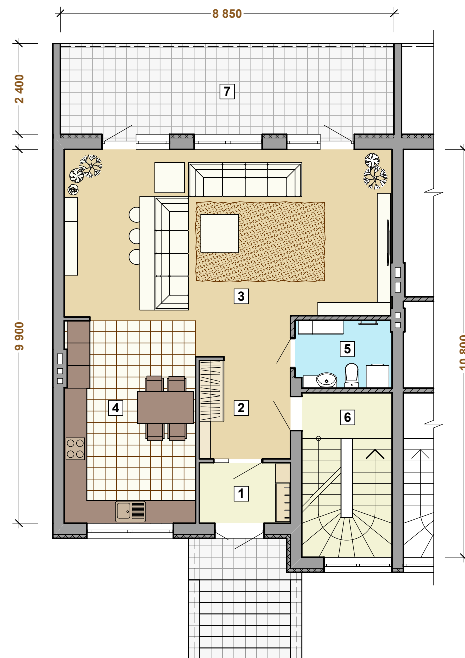
ПЕРВЫЙ ЭТАЖ
