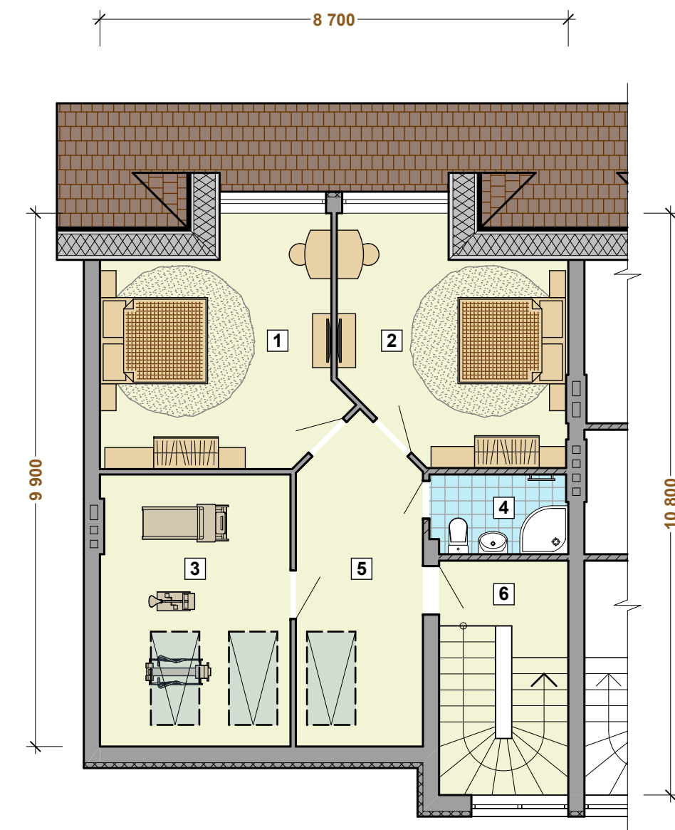
МАНСАРДНЫЙ ЭТАЖ
