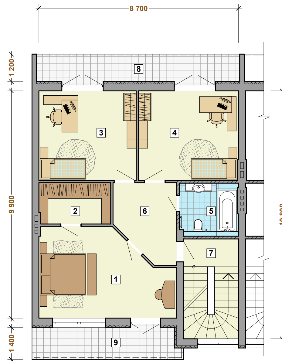
ВТОРОЙ ЭТАЖ
