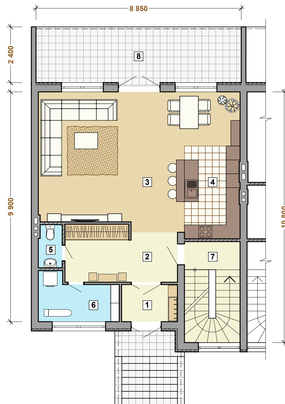
ПЕРВЫЙ ЭТАЖ
